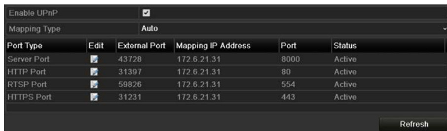
図 11.25 UPnP™設定終了-オート
