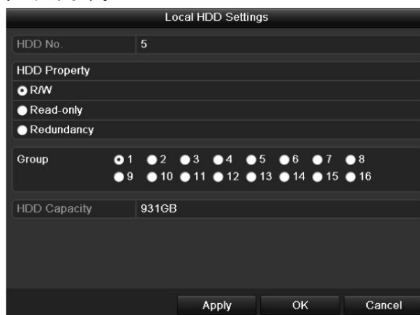
図 13.17 HDD プロパティの設定
