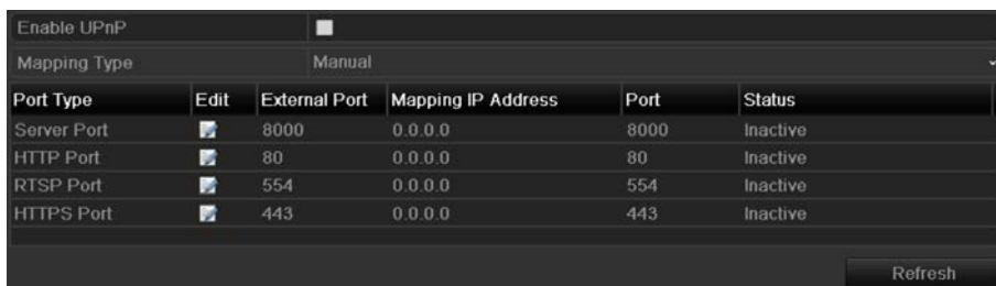
図 11.24 UPnP™設定インターフェイス
