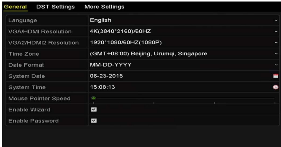
図 16.2 一般設定インターフェイス (DS-9600NI-I8)
