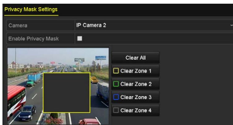
図 14.3 プライバシーマスクエリアの設定
